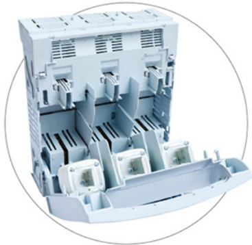
开启结构图
