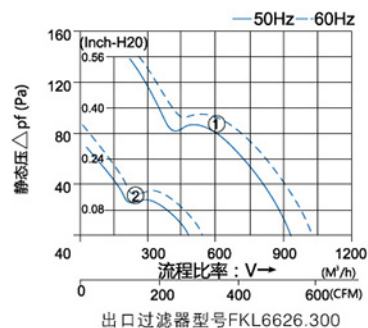
功率特性曲线 FKL 6626....
