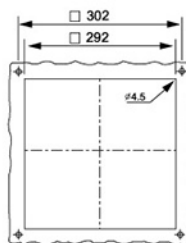
安装剖面 FKL 6626....
