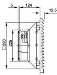
风扇及过滤器 FKL 6626.230
