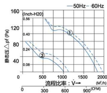
功率特性曲线 FKL 6626....
