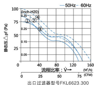
功率特性曲线 FKL 6623....
