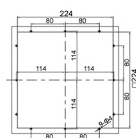
安装剖面 FKL 5525-200....
