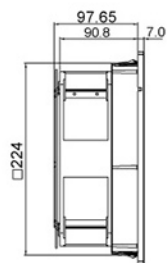
风扇及过滤器 FKL 5525-200.230
