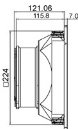
风扇及过滤器 FKL 5525-162.230
