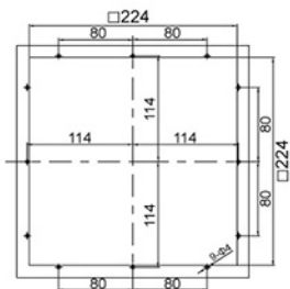
安装剖面 FKL 5525-162....
