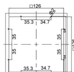
安装剖面 FKL 5522....
