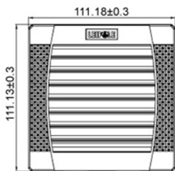
风扇及过滤器 FKL 5521....
