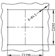
风扇及过滤器 FK9926.230-260.NO (常开)
