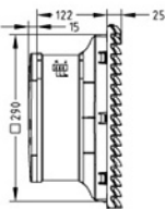
出口过滤器 FK 9926.300
