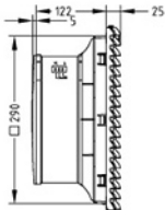
风扇及过滤器 FK 9926.230
