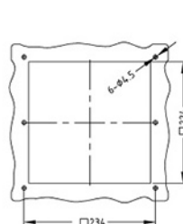
风扇及过滤器 FK9925.230-162.NO (常开)
