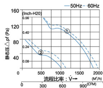
功率特性曲线 FK 7726....
