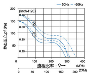
功率特性曲线 FB 9805....
