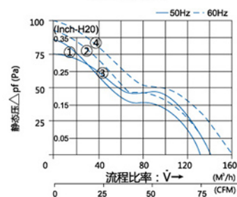
功率特性曲线 FB 9804....
