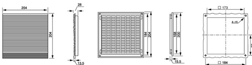
外形尺寸
