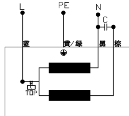
接线图
