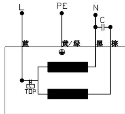
接线图
