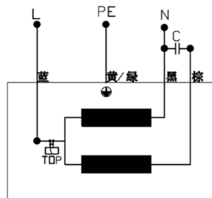
接线图
