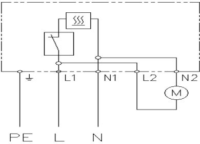
电路原理图如下:
