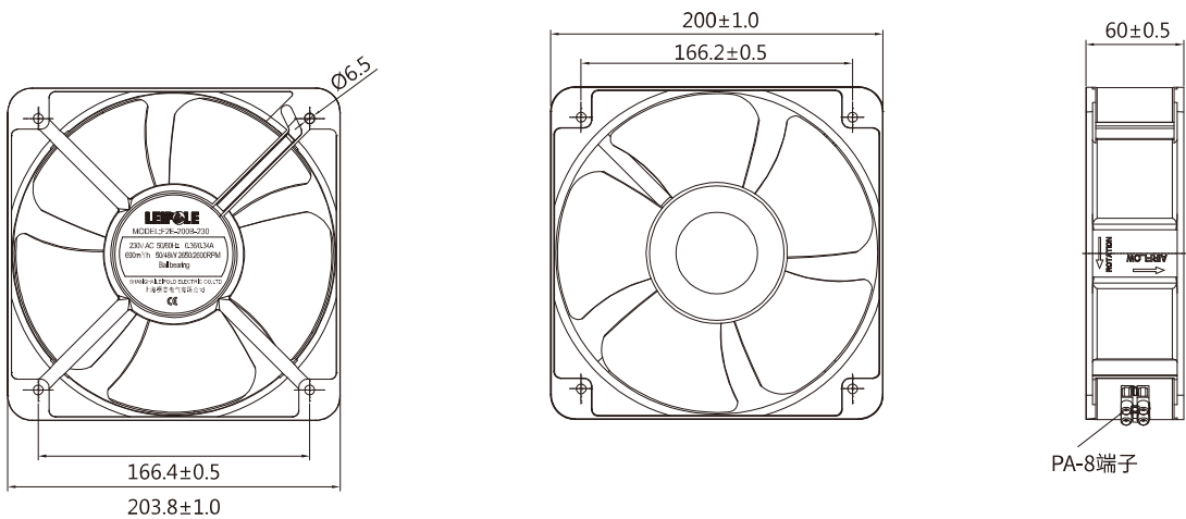
外形尺寸
