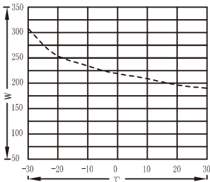
JRQFS200曲线图
