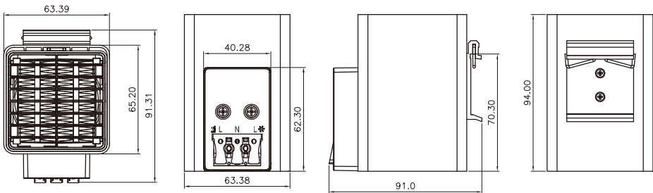
外形尺寸
