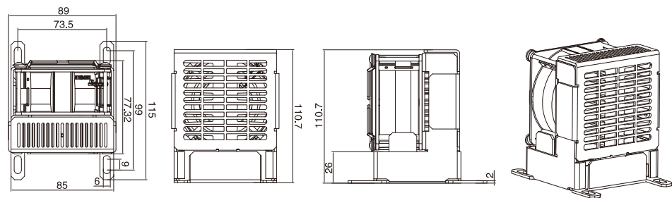
外形尺寸
