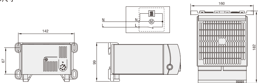
外形尺寸
