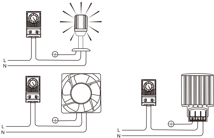
安装图示
