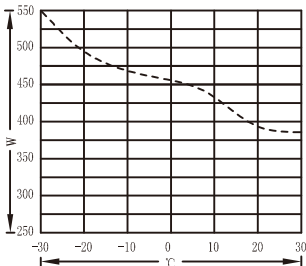
JRQFS400曲线图
